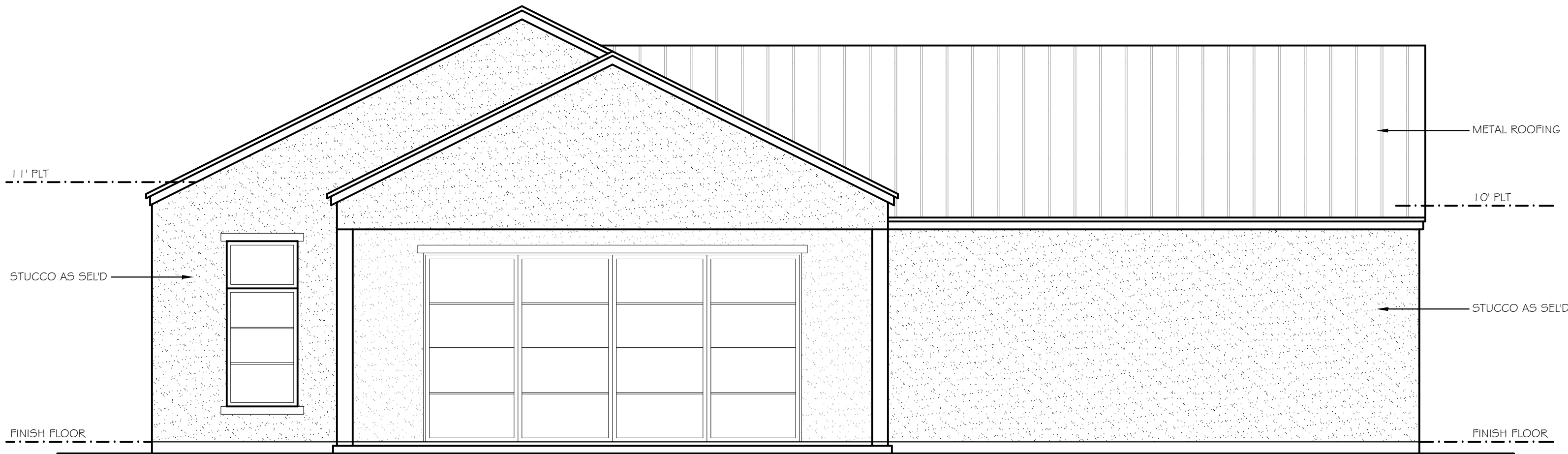
RIGHT ELEVATION
